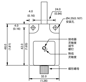
光纤传感器侧视图
