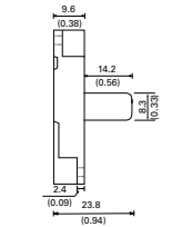
光纤传感器侧视图
