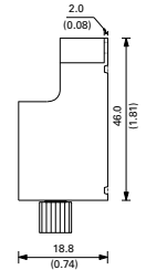
光纤传感器侧视图
