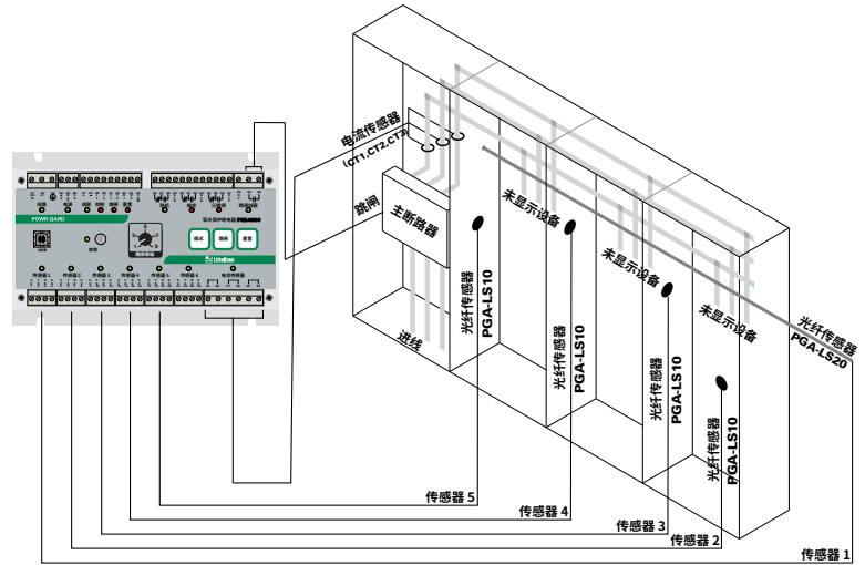
PGA-LS20 10米 (8米有效) PGA-LS25 8米 (5米有效) PGA-LS30 20米 (18米有效)
