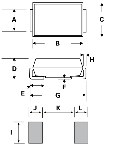
DO-214AC (SMA)
