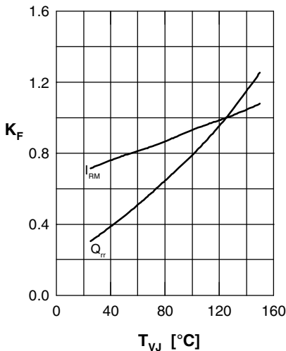
Fig. 4 Typ. dynamic parameters K_F , I_{RM} , Q_{rr} versus T_{VJ}
