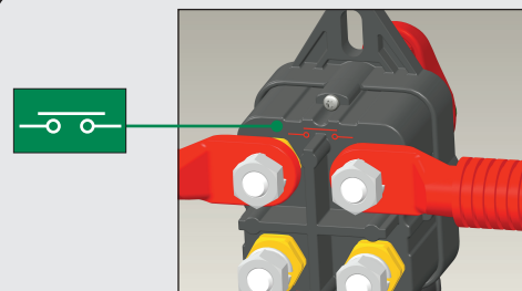
D1 Orientamento staccabatteria Battery disconnect orientation
