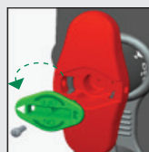
B4 Ruotare l'inserto verde di 180° e fissarlo alla maniglia Rotate the green insert 180° and screw it to the handle
