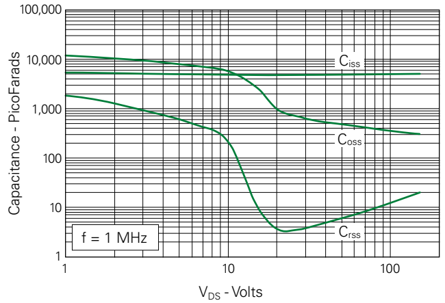
Fig. 12. Capacitance
