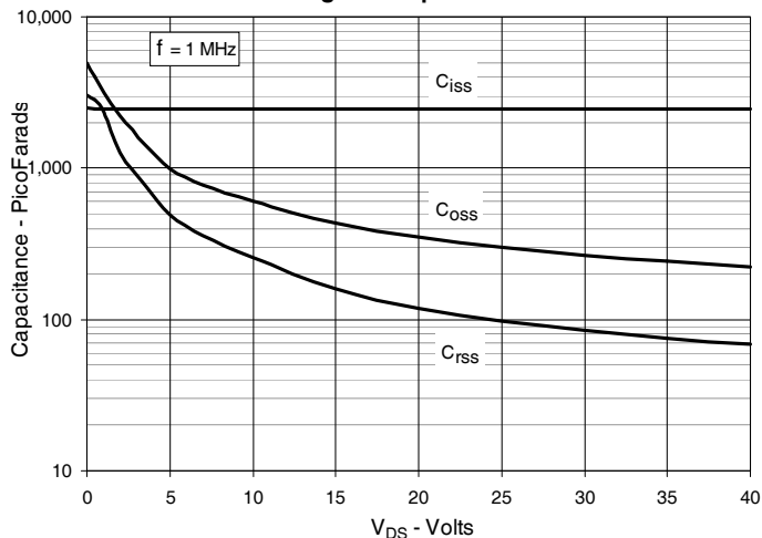
Fig. 12. Capacitance
