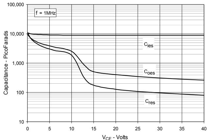
Fig. 8. Capacitance
