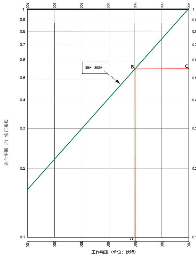
图 20: 完全熔断 I 2 t 修正系数曲线
