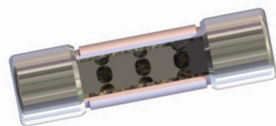
图 11b: 圆柱或金属箍样式熔断器
