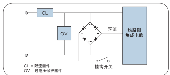
图2 调制解调器接口
